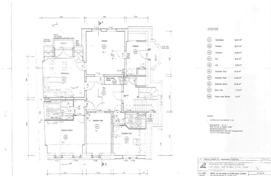
GrundrissDG
